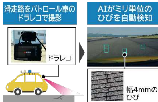
ドライブレコーダーを活用した滑走路点検
